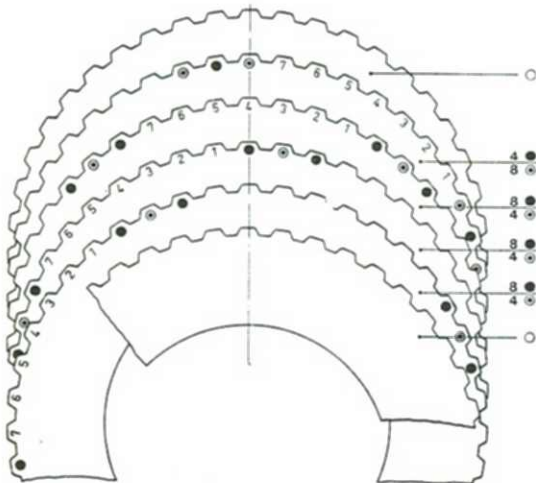
Fig. 19 Grandezza apparecchio: 29
