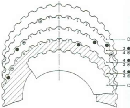
Fig. 17 Grandezza apparecchio: 19 e 24 Nella grandezza 24 manca la lamella tratteggiata
